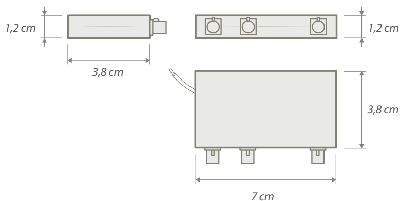
Dimensions / Dimensioni
